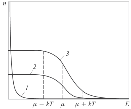
Общий вид статистик Бозе–Эйнштейна (1), Ферми–Дирака (2) и обобщенной статистики (3)
